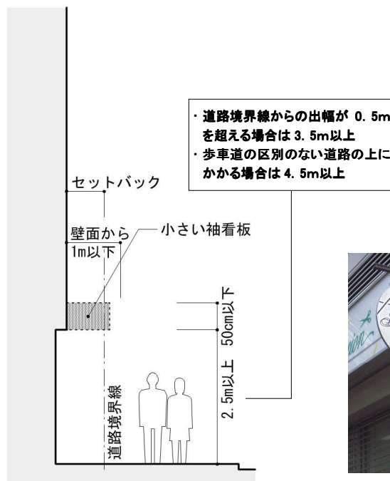
図3：上下寸法50cm×幅1m以下の袖看板
