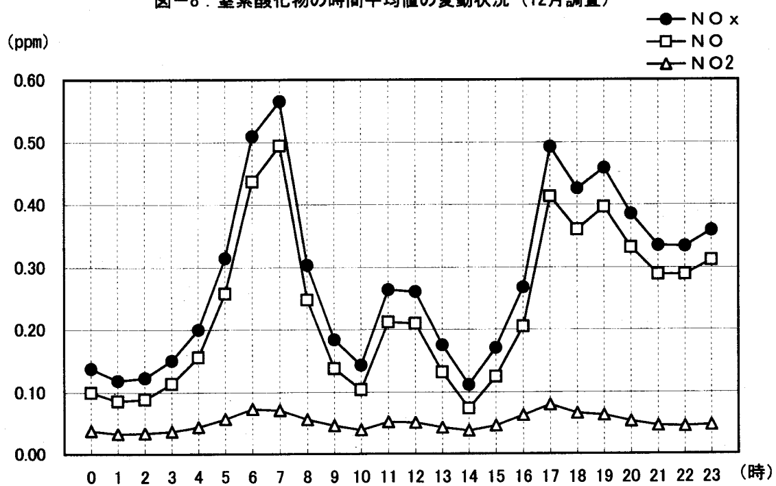
図-8：窒素酸化物の時間平均値の変動状況（12月調査）
