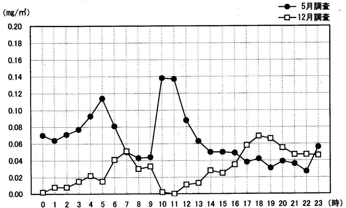
図-4：浮遊粒子状物質の時間平均値の変動状況（季節別）
