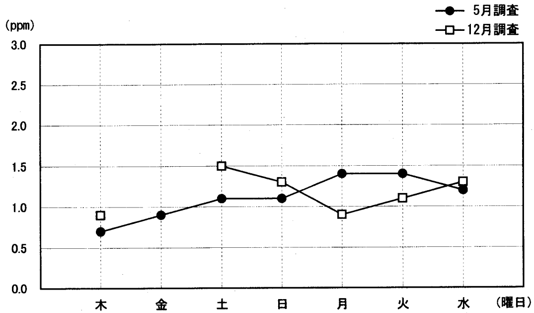
図-1：一酸化炭素の日平均値の変動状況（季節別）
