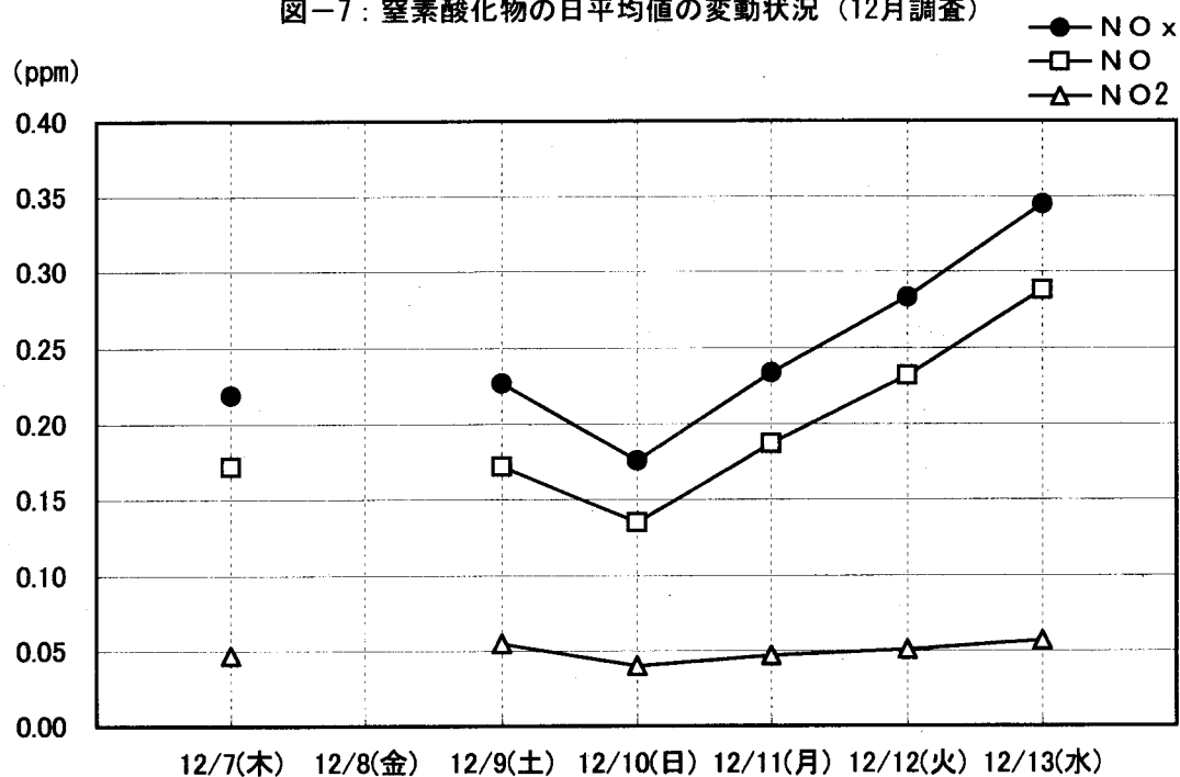
図-7：窒素酸化物の日平均値の変動状況（12月調査）
