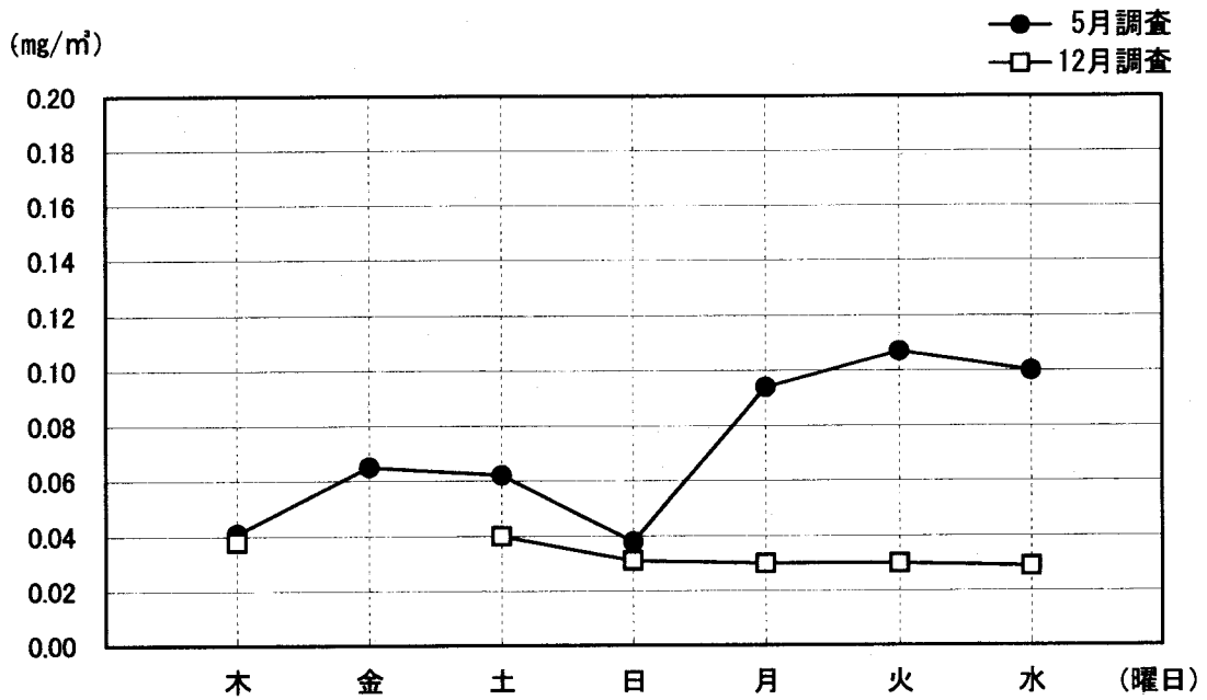
図-3：浮遊粒子状物質の日平均値の変動状況（季節別）
