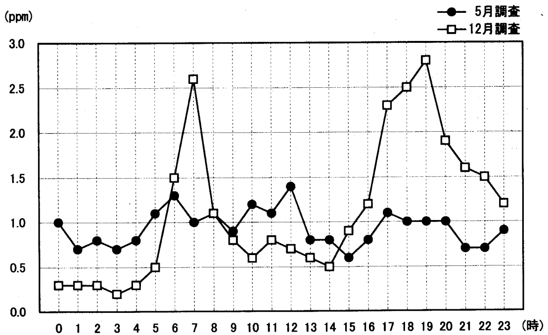
図-2：一酸化炭素の時間平均値の変動状況
