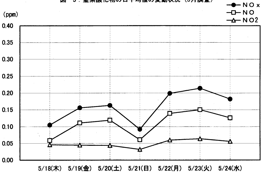
図-5：窒素酸化物の日平均値の変動状況（5月調査）
