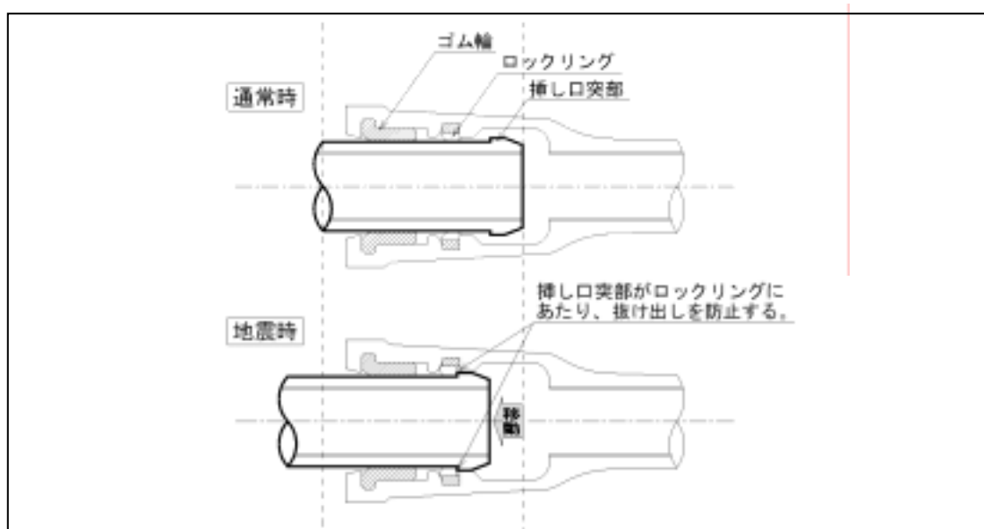
図 11 耐震継手（離脱防止機能）のイメージ（通常時と地震時、NS 型の例）
