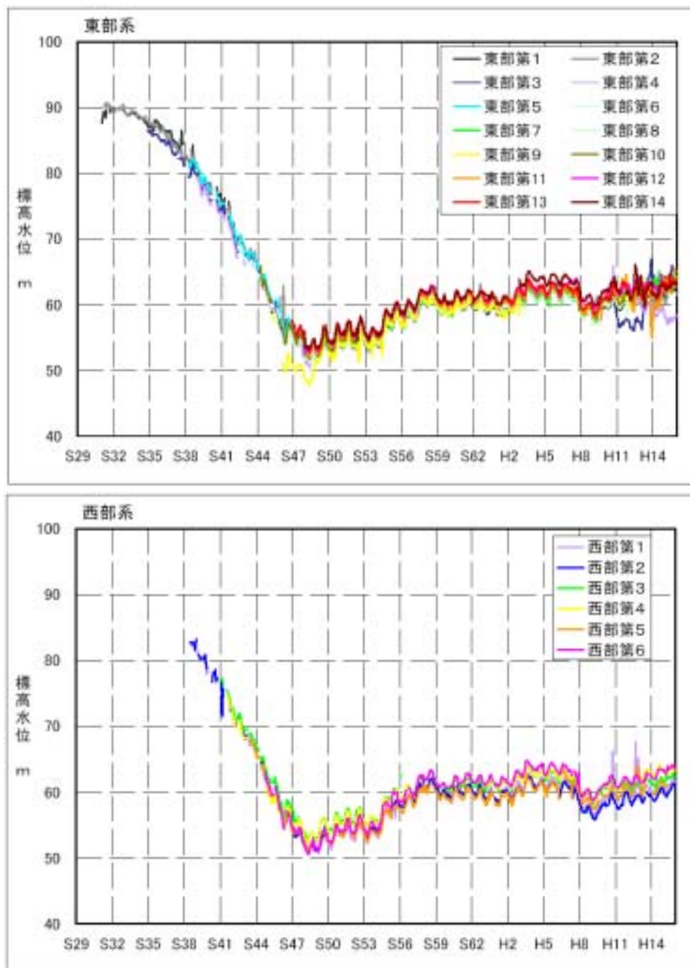
図6 昭島市の水源井戸における水位 (昭島市周辺地下水流動実態調査報告書より)
