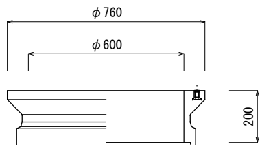
上部ブロック (200A)
