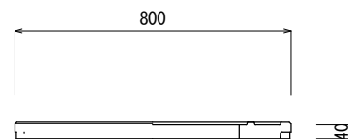
底版
