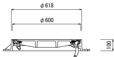
鉄蓋
