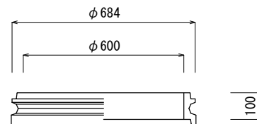
中部ブロック (100B)
