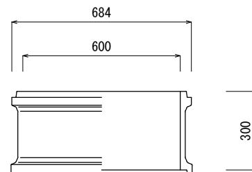
中部ブロック (300B)
