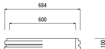
下部ブロック (100C)
