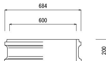
下部ブロック (200C)
