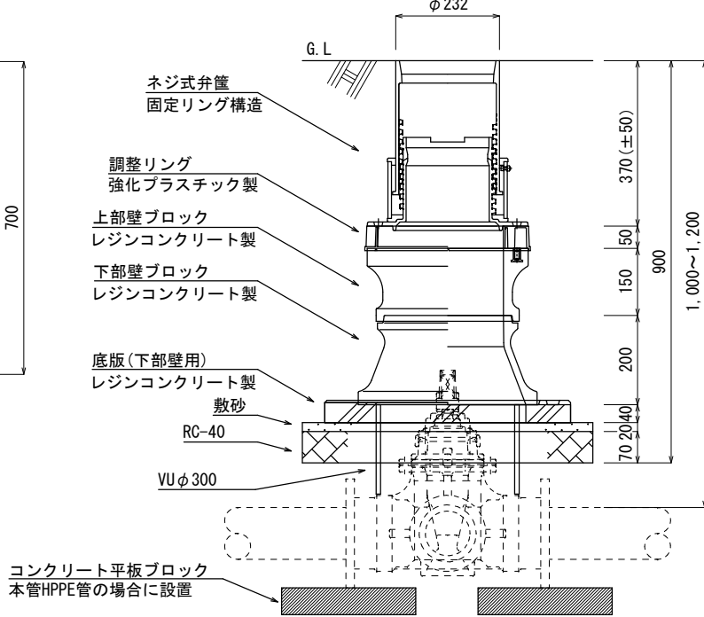
側面図 Cタイプ
