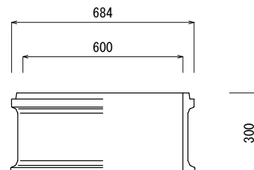
下部ブロック (300C)
