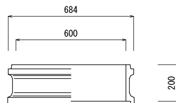
中部ブロック (200B)
