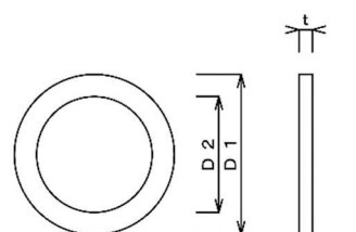
付図1 メーターパッキン
