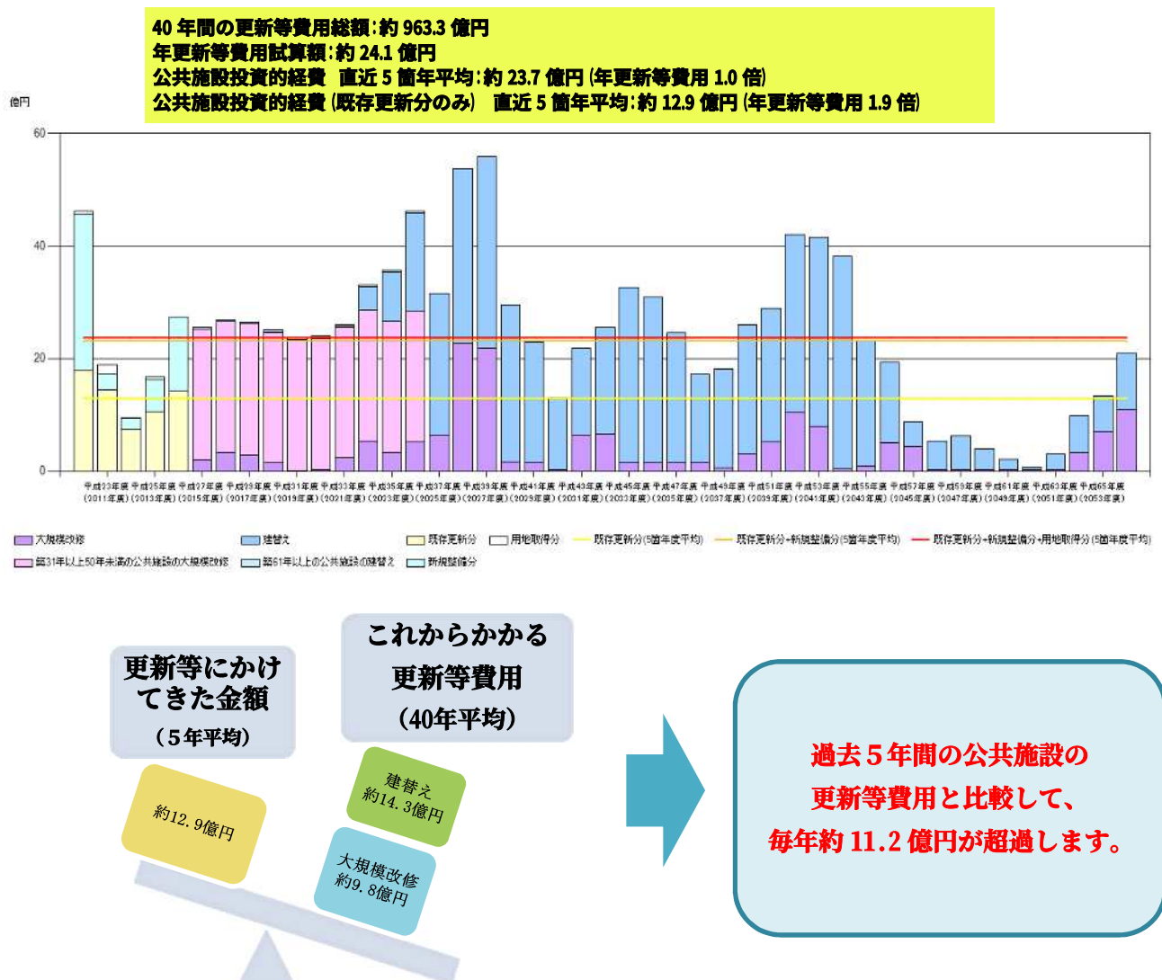
図 1-5-12 公共施設の更新等費用試算
