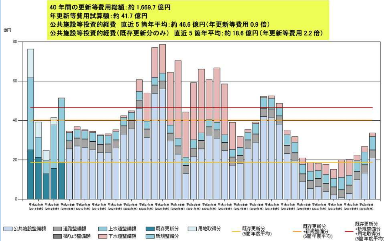
公共施設等（公共施設とインフラ）の更新等費用試算のグラフ
