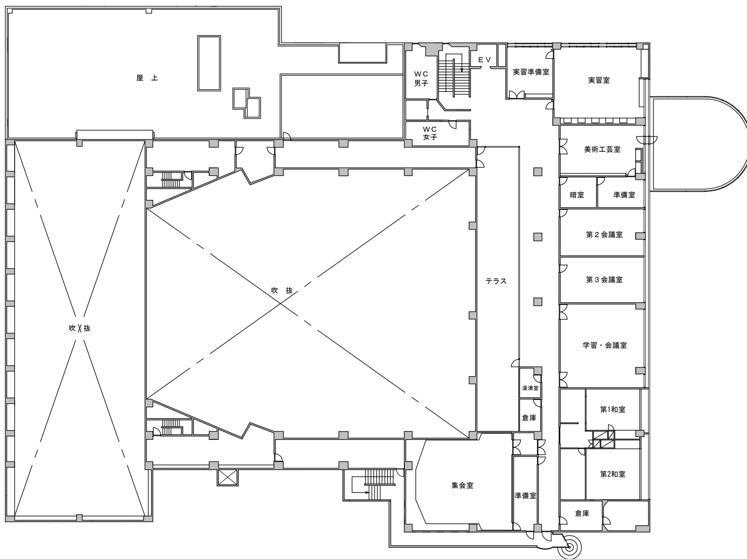
昭島市民会館・公民館 3 F 平面図 S = 1 / 4 0 0
