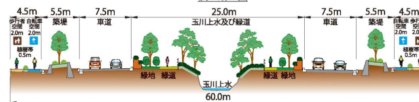
横断図
