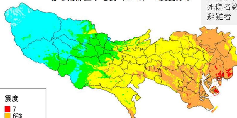
都心南部直下地震（M7.3）の震度分布
