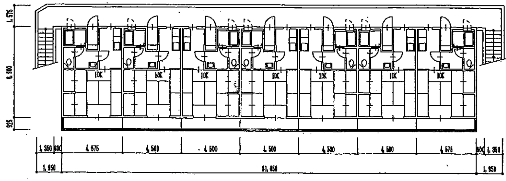
2階平面図
