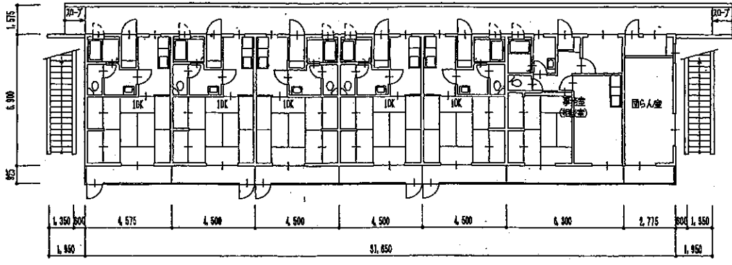
1階平面図
