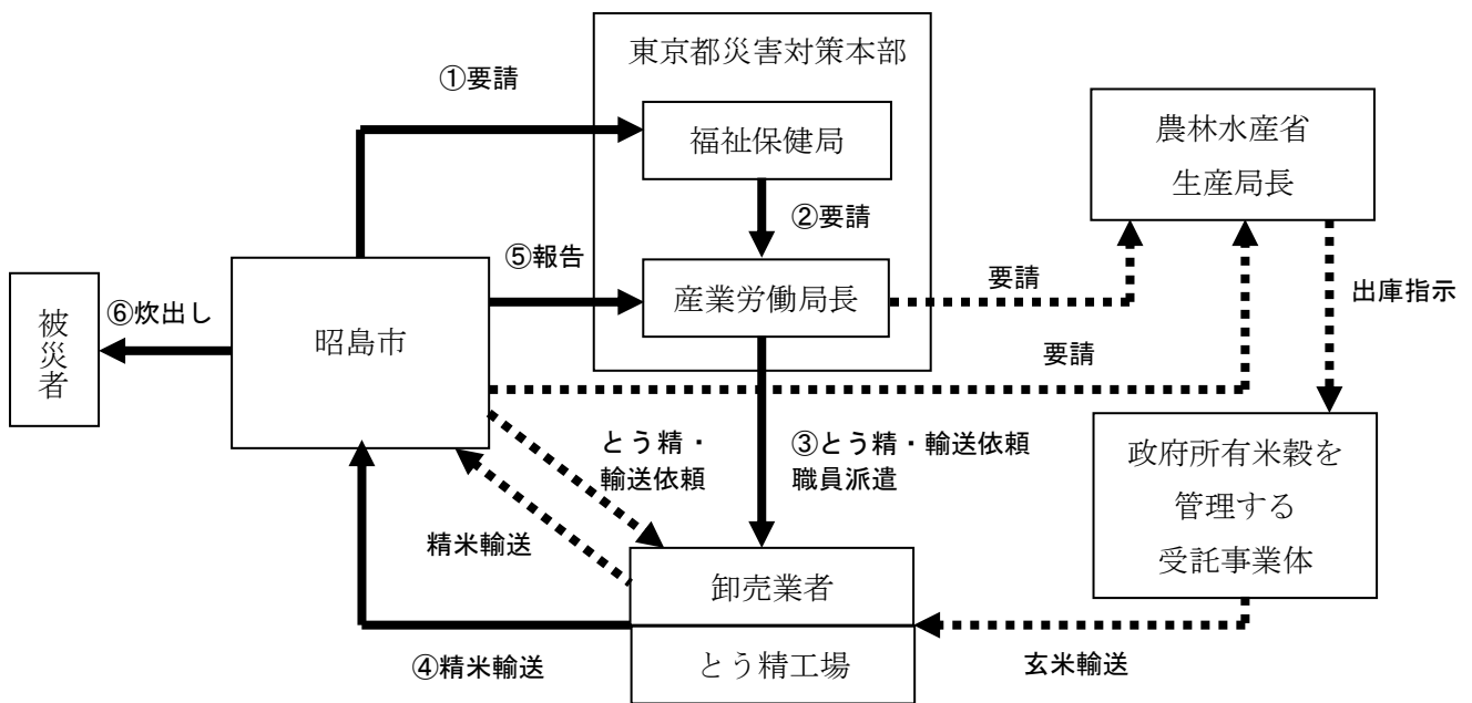
【米穀の調達フロー図】
